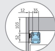
Altura colgador. Hanger height. Hauteur de l'accroche.
